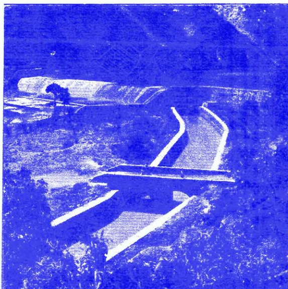
↑ 這座弓形空心坝，是紅旗渠上的一座特殊建築物。它使河水經坝頂順流而下，渠水却通過坝心，流向南山，很好地解決了渠水和河水交叉的矛盾。那些資產階級反動學術“權威”們想也不敢想的奇跡，林縣的貧下中農創造出來了。
