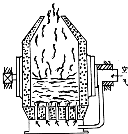
柏塞麥煉鋼爐
